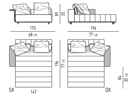
CHAISE-LONGUE CM 175X196
