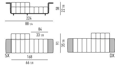
DIVANO OPEN CM 224 - SCHIENALE CM 84 OPEN SOFA CM 224 - BACKREST CM 84
