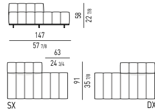
ELEMENTO PENISOLA CM 147 - SCHIENALE CM 84 OPEN-END ELEMENT CM 147 - BACKREST CM 84
