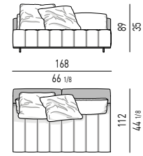
SOFÁ CM 168 - N° 2 SCHIENALI CM 84 SOFÁ CM 168 - N° 2 BACKRESTS CM 84
