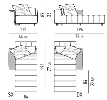
CHAISE-LONGUE CM 112X196
